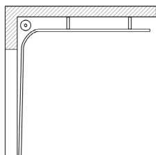
Рис. 1. Стандартный монтаж
