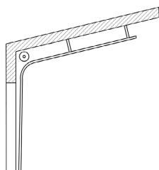
Рис. 7. Наклонный монтаж
