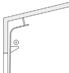
Рис. 9. Наклонный высокий монтаж с нижним расположением вала
