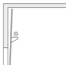
Рис. 6. Вертикальный монтаж с нижним расположением вала
