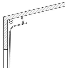
Рис. 8. Наклонный высокий монтаж с верхним расположением вала
