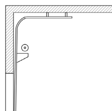
Рис. 3. Высокий монтаж с нижним расположением вала
