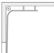
Рис. 4. Высокий монтаж с верхним расположением вала
